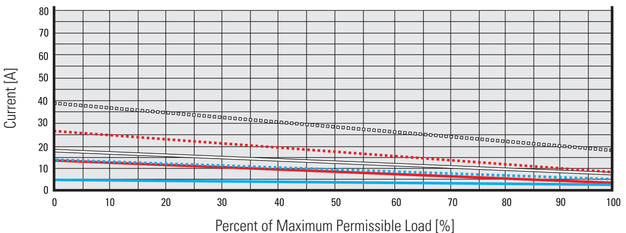
12 Vdc Actuators
